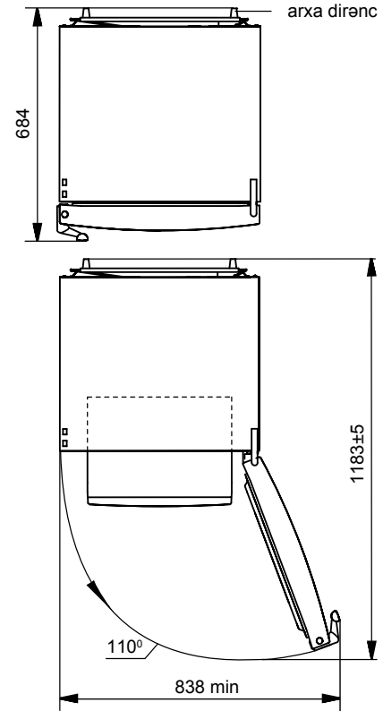
Şəkil 2 – Dondurucu (yuxarıdan görünüşü)
