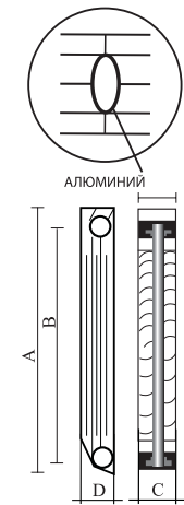
Чертежи радиатора в разрезе
