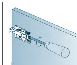
Притягивание навеса к
