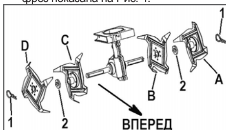
Рис. 4 Установка фрез
