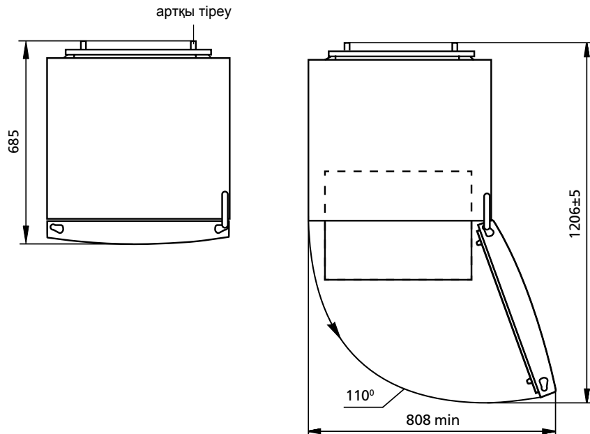
2 сурет — Тоңазытқыш (жоғарыдан көрінетін түр)
