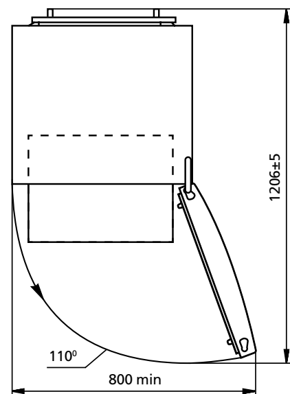
Şəkil 2 — Soyuducu (üstədən görünüşü)
