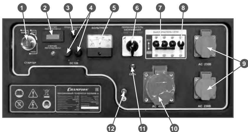
Рис. 3 Панель управления
