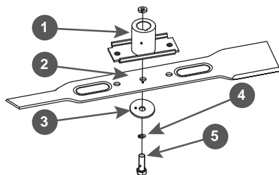
Рис. 18 Обслуживание ножа
