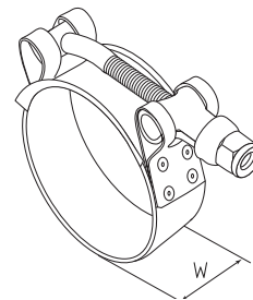
Конструкция силовых хомутов T-bolt ST/W2
