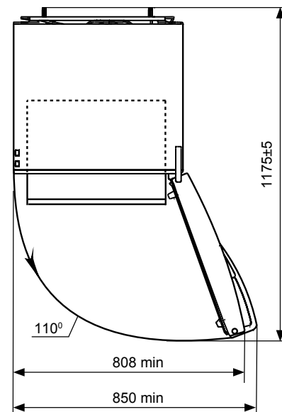
2-сурет – Тоңазытқыш (жоғарыдан қарағандағы түрі)
