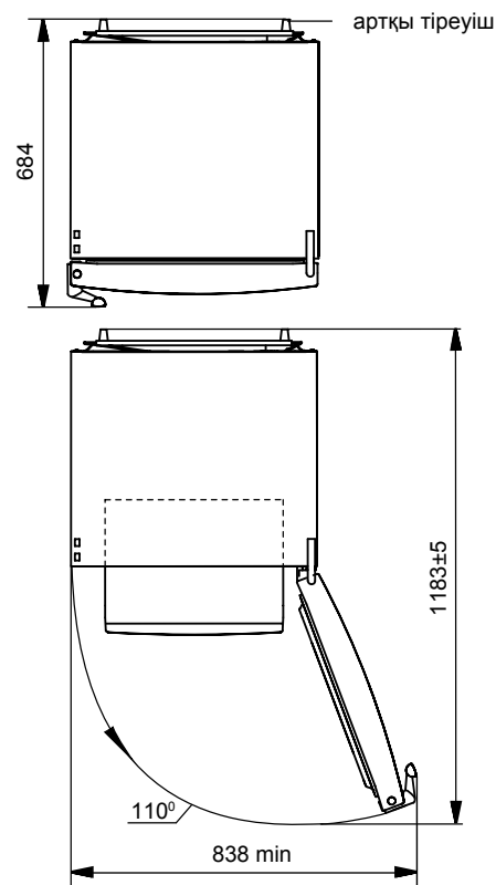
2-сурет – Мұздатқыш (жоғарыдан қарағандағы түрі)
