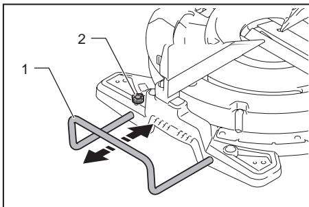
► 1. Holder 2. Screw
