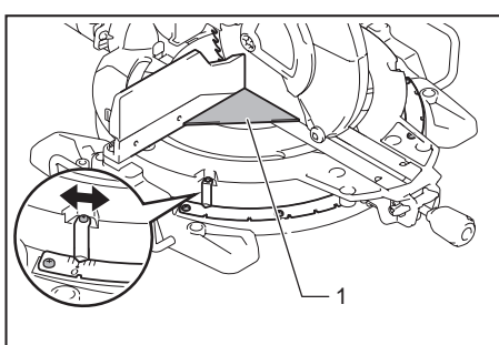
► 1. Règle triangulaire
