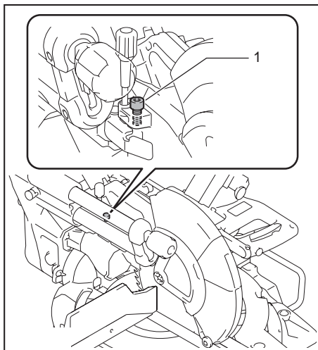
► 1. Adjusting bolt
