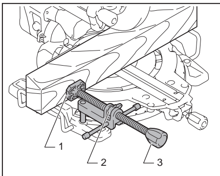
► 1. Vise plate 2. Vise nut 3. Vise knob
