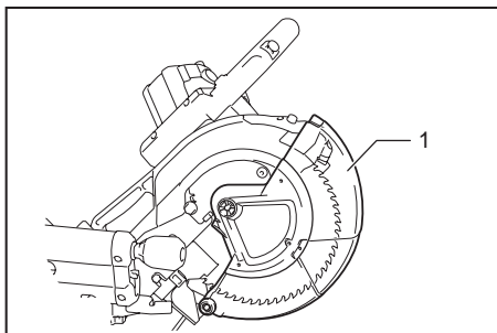
► 1. Blade guard
