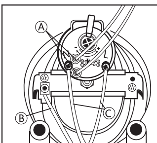
Автоклавный фланец
