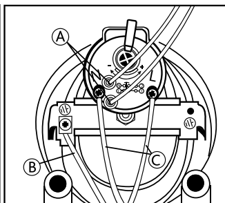
Автоклапный фланец
