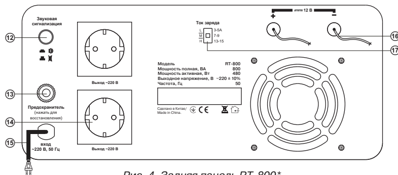
Рис. 4. Задняя панель RT-800*
