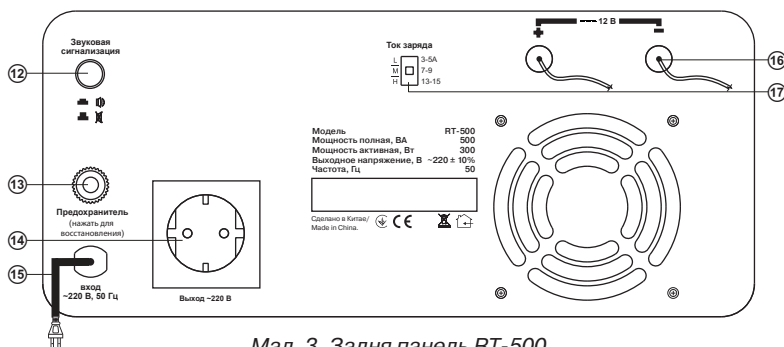
Мал. 3. Задня панель RT-500
