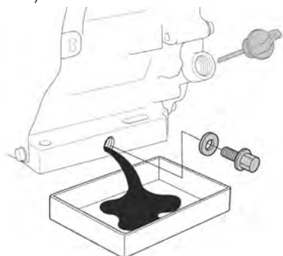
Рис. 15 Замена масла в двигателе
