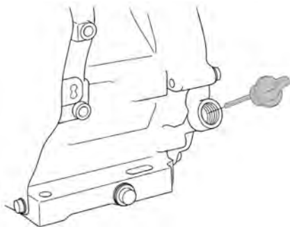
Рис. 8 Крышка-щуп маслозаливной горловины
