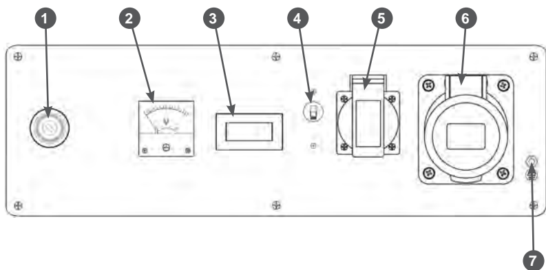
Рис. 3 Панель управления
