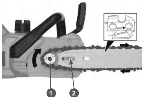
Рис. 3. Установка цепи
