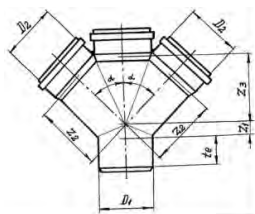
Рис 4. Крестовина одноплоскостная
