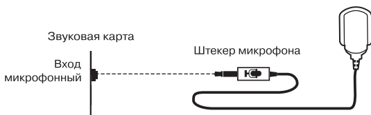
Рис. 1. Схема подключения
