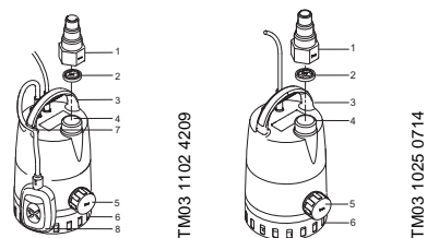
Рис. 1 Разрез насоса Unilift CC
