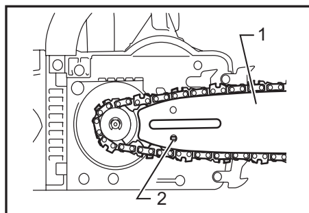
► 1. Стержень направляющей 2. Отверстие
