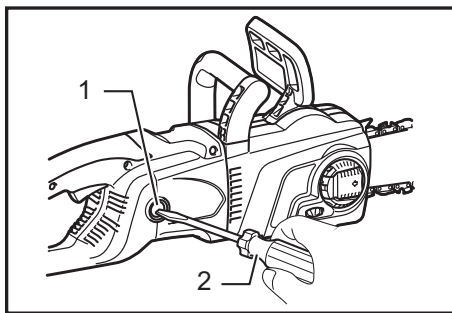
► 1. Колпачок держателя щетки 2. Отвертка
