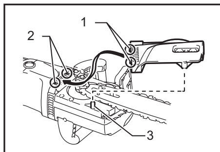
► 1. Крючок 2. Отверстие 3. Штифт
