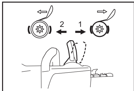
1. Тормоз цепи включен 2. Тормоз цепи выключен
