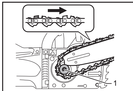
► 1. Звездочка
