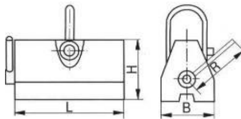
Рис.2 - Габаритные размеры магнитного захвата
