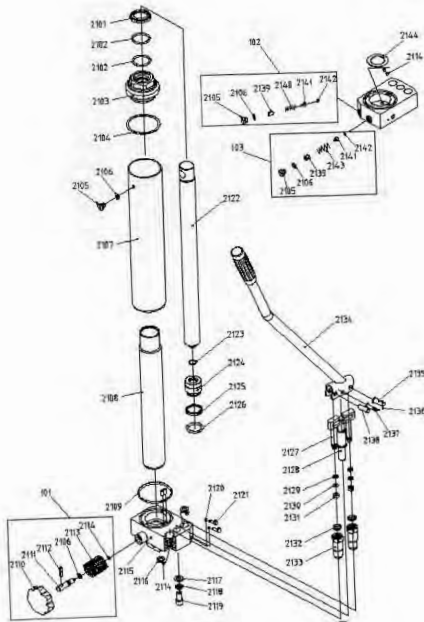
Схема 4. Гидравлический цилиндр.
