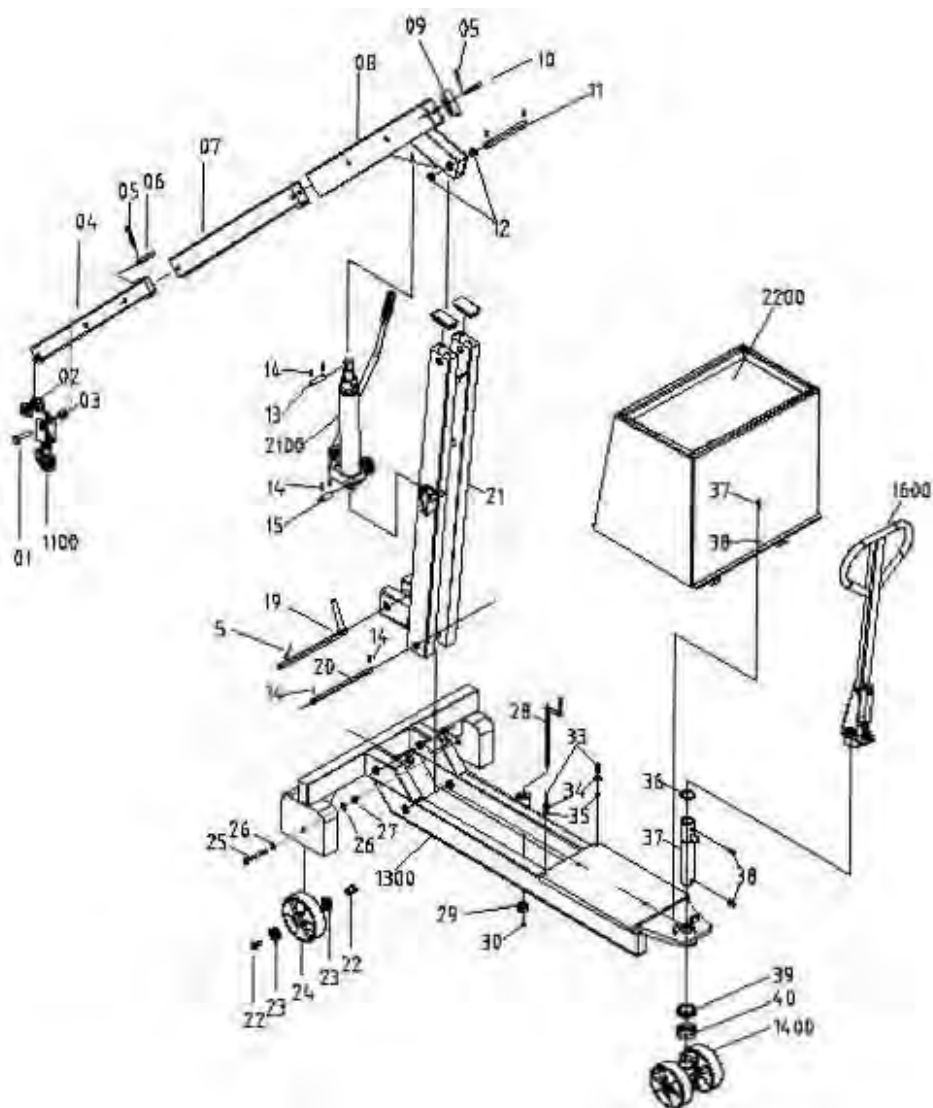
Схема 1. Кран с противовесом (каталог запасных частей).
