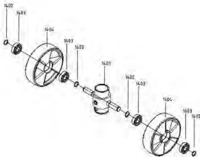
Схема 5. Колеса.
