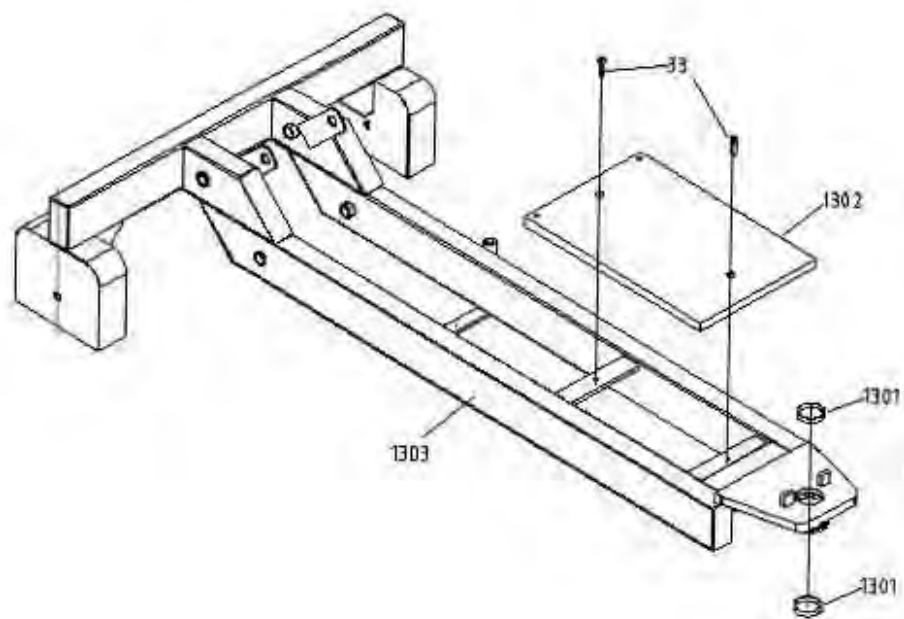
Схема 3. Шасси.
