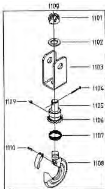
Схема 2. Крюк.
