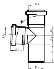
Рисунок 13. Тройники
