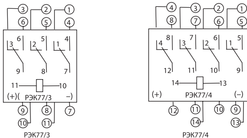
Рисунок 2. Схемы подключения
