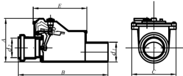
Рисунок 14. Обратные клапана
