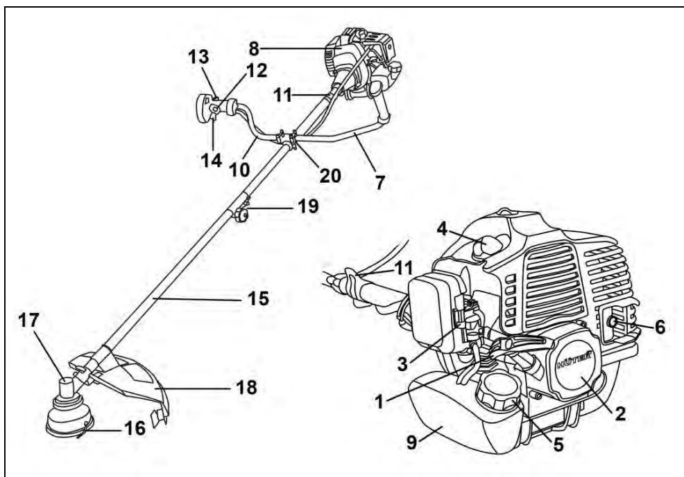
Рис. 1. Общий вид.
