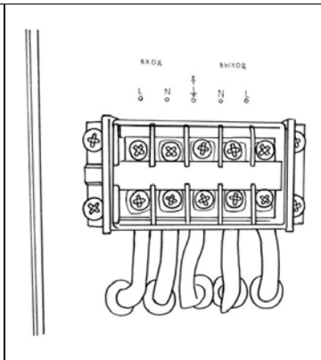
Рис. 6. Схема подключения
