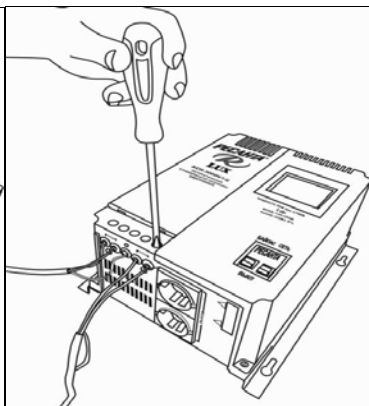
Рис. 8. Подключение нагрузки
