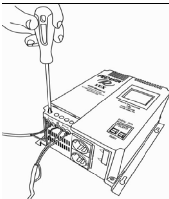
Рис. 7. Подключение стабилизатора
