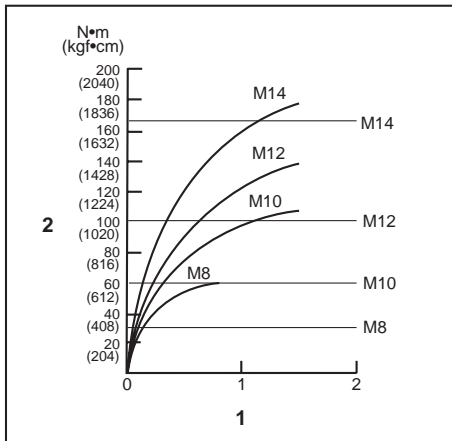
1. Koha e shtrëngimit (sekonda) 2. Forca e shtrëngimit
