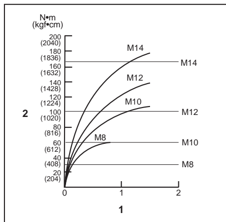
1. Čas privijanja (s) 2. Zatezni moment
