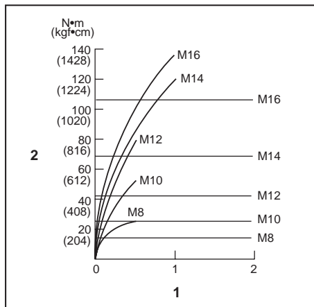
1. Час затягування (с) 2. Момент затягування
