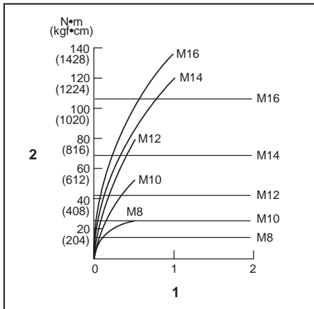
1. Koha e shtrëngimit (sekonda) 2. Forca e shtrëngimit
