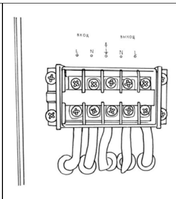
Рис. 6. Схема подключения
