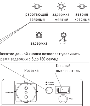
Рис. 2 Внешний вид стабилизатора W-500
