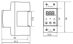
Рисунок 1. Габаритные и установочные размеры реле напряжения серии PH 2, мм
