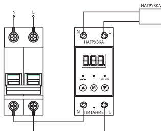
Рисунок 2. Схема подключения реле
