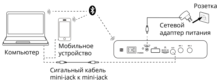
Рис.3. Схема подключения
