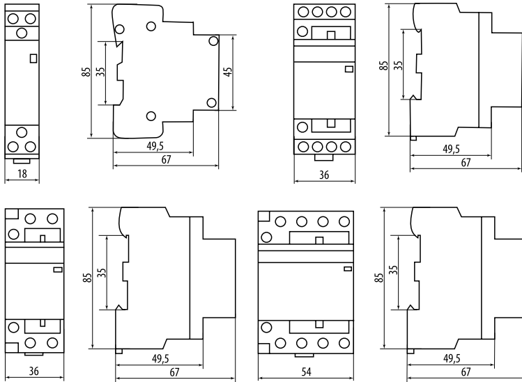
Рисунок 1. Габаритные размеры
