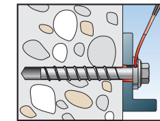
Empfohlen für die Anwendungen nach der Seismischen Leistungskategorie C1: Der Spalt zwischen Schraubenschaft und Anbauteil kann mit Mörtel verfüllt sein; Druckfestigkeit \geq 50 \text{ N/mm}^2 z.B.: FIS V, FIS EM Plus, FIS HB oder FIS SB.
