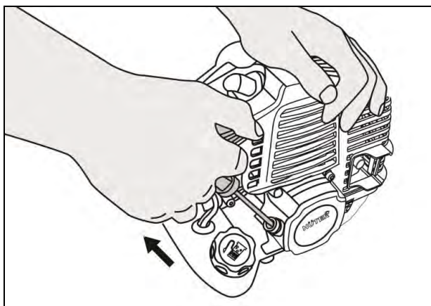
Рис. 25. Запуск двигателя
