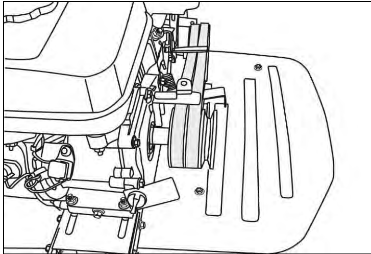
Рис. 49. Правильное положение приводных ремней
