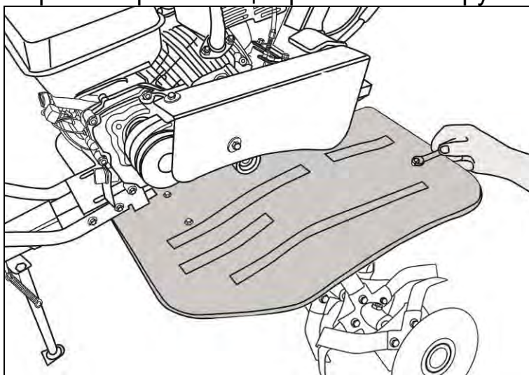
Рис. 15. Фиксация крыльев
