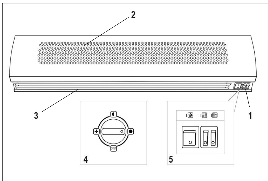
Рис. 1. Общий вид
