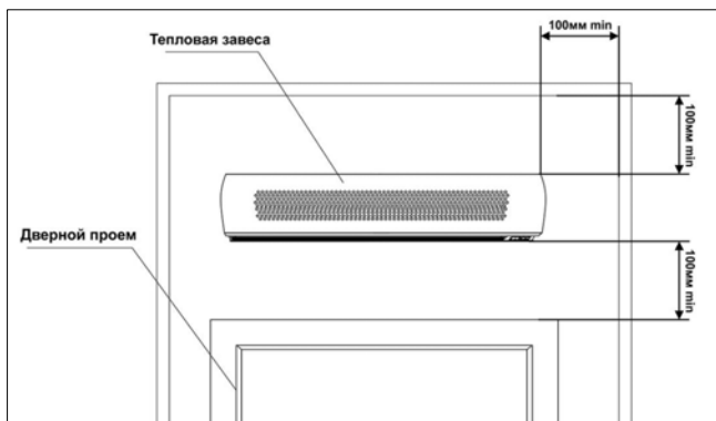
Рис. 3. Расположение завесы
