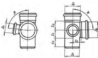
Рис 5.1. Крестовина двухплоскостная
