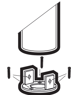
Рис.6 Схема крепления светильника PGB 04-800 к опорной поверхности
