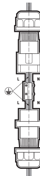
Рис.7 Схема подключения светильника к электросети
