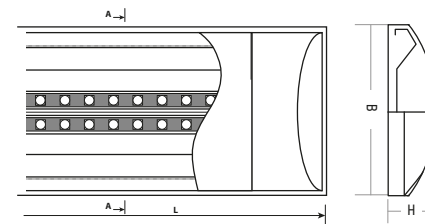
Рис. 2 Светильники PPO-03 1500
