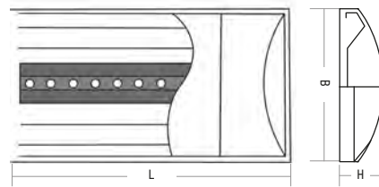
Рис. 1 Светильники PPO-03 600 / PPO-03 1200
