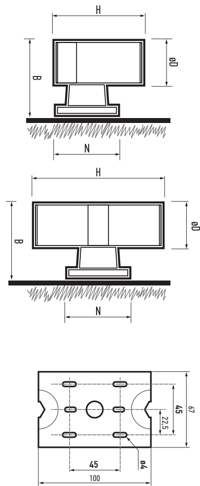
Рис. 1 Одностороннее свечение
