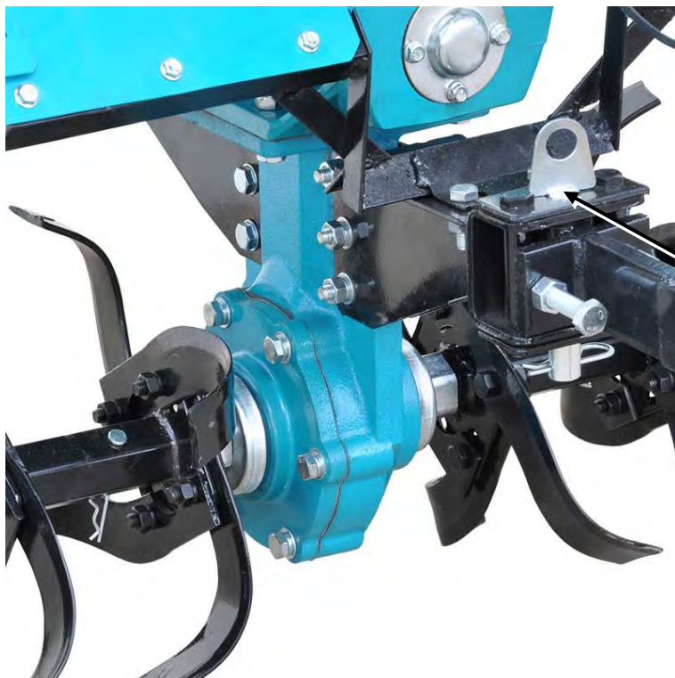
Стопорный палец
