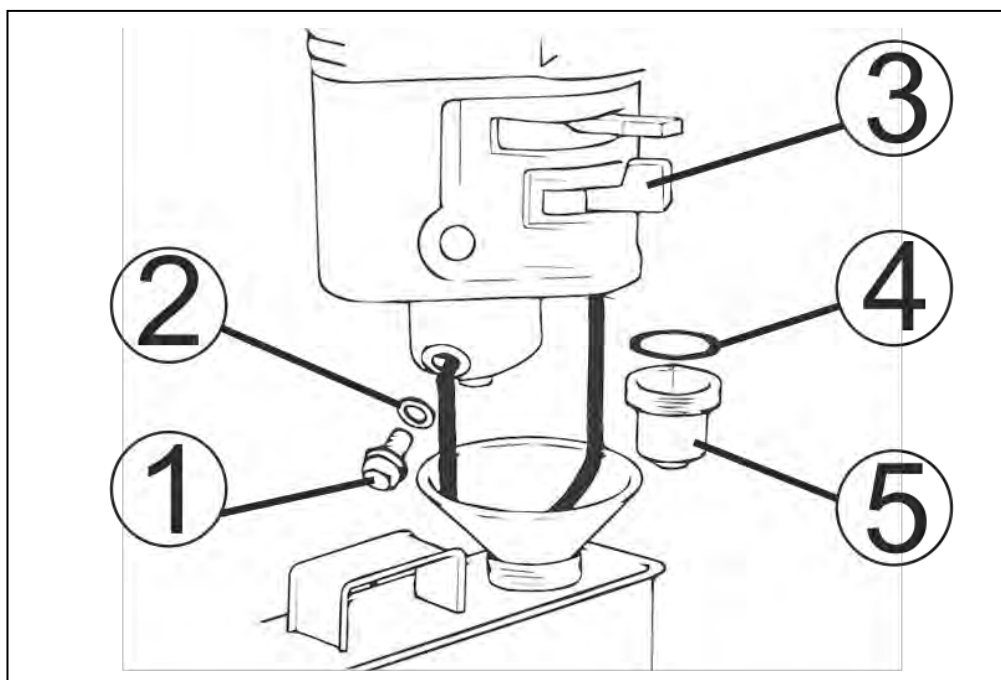
Рис. 18. Обслуживание фильтра-отстойника.
