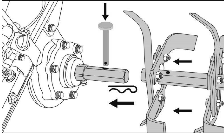
Рис. 6. Установка фрезы
