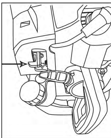
Рис. 9 Открытие воздушной заслонки
