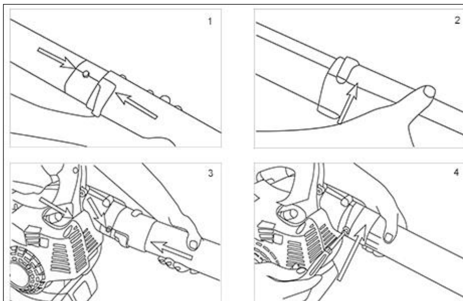
Рис. 2 Сборка бензиновой воздуходувки
