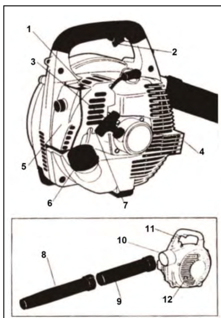
Рис. 1 Общий вид
