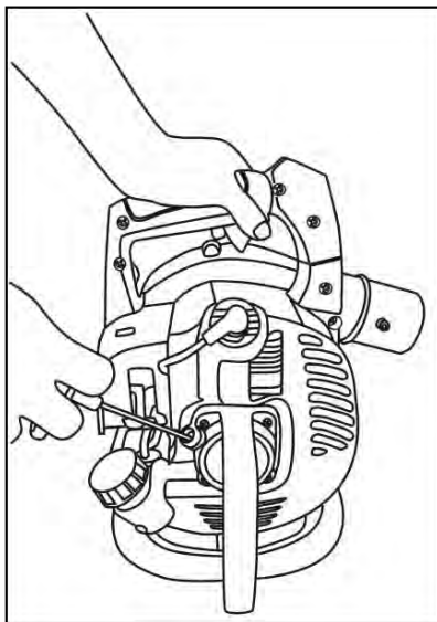
Рис. 12 Запуск двигателя
