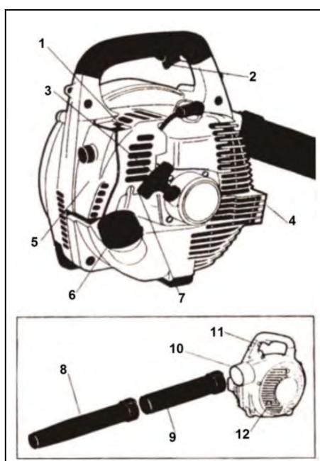
Рис. 1 Общий вид
