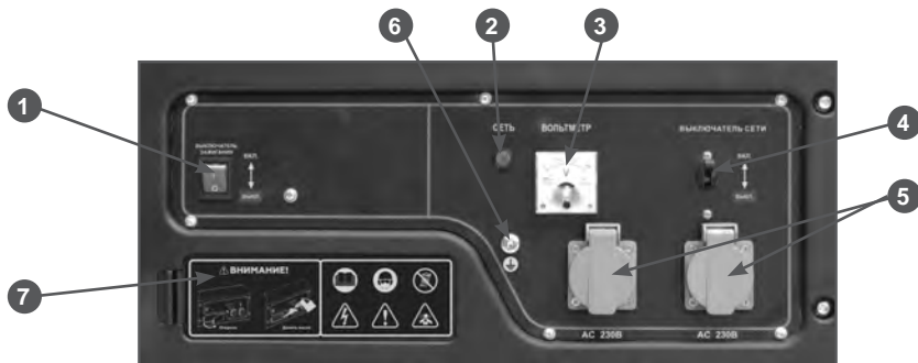
Рис. 3 Панель управления
