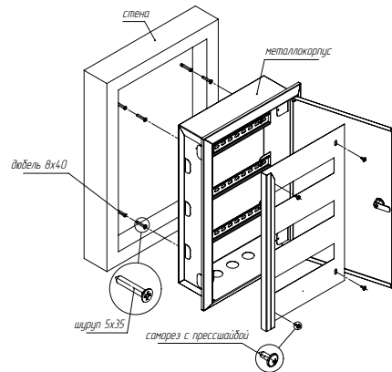
Рис. 1. Схема монтажа
